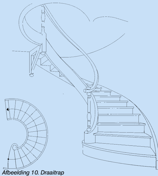
Afbeelding 10. Draaitrap
