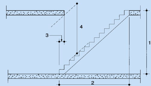
Afbeelding 6. - 1. Verdiepingshoogte, 2. traplengte, 3. insprong en 4. vrije hoogte.
