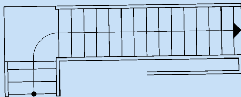
Afbeelding 7. Rechte trap met kwartbordes
